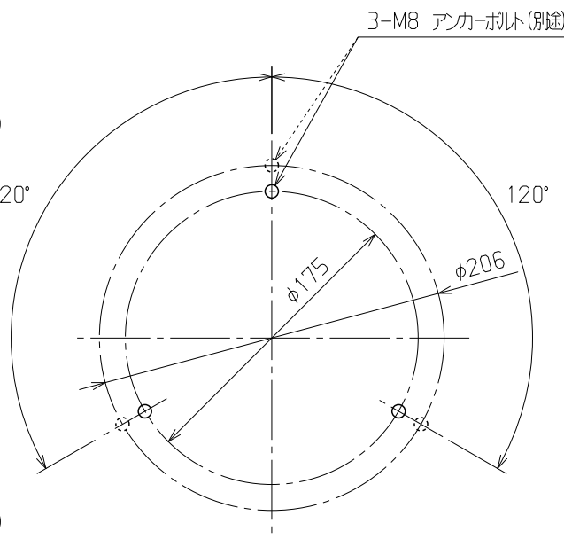
取付寸法図
